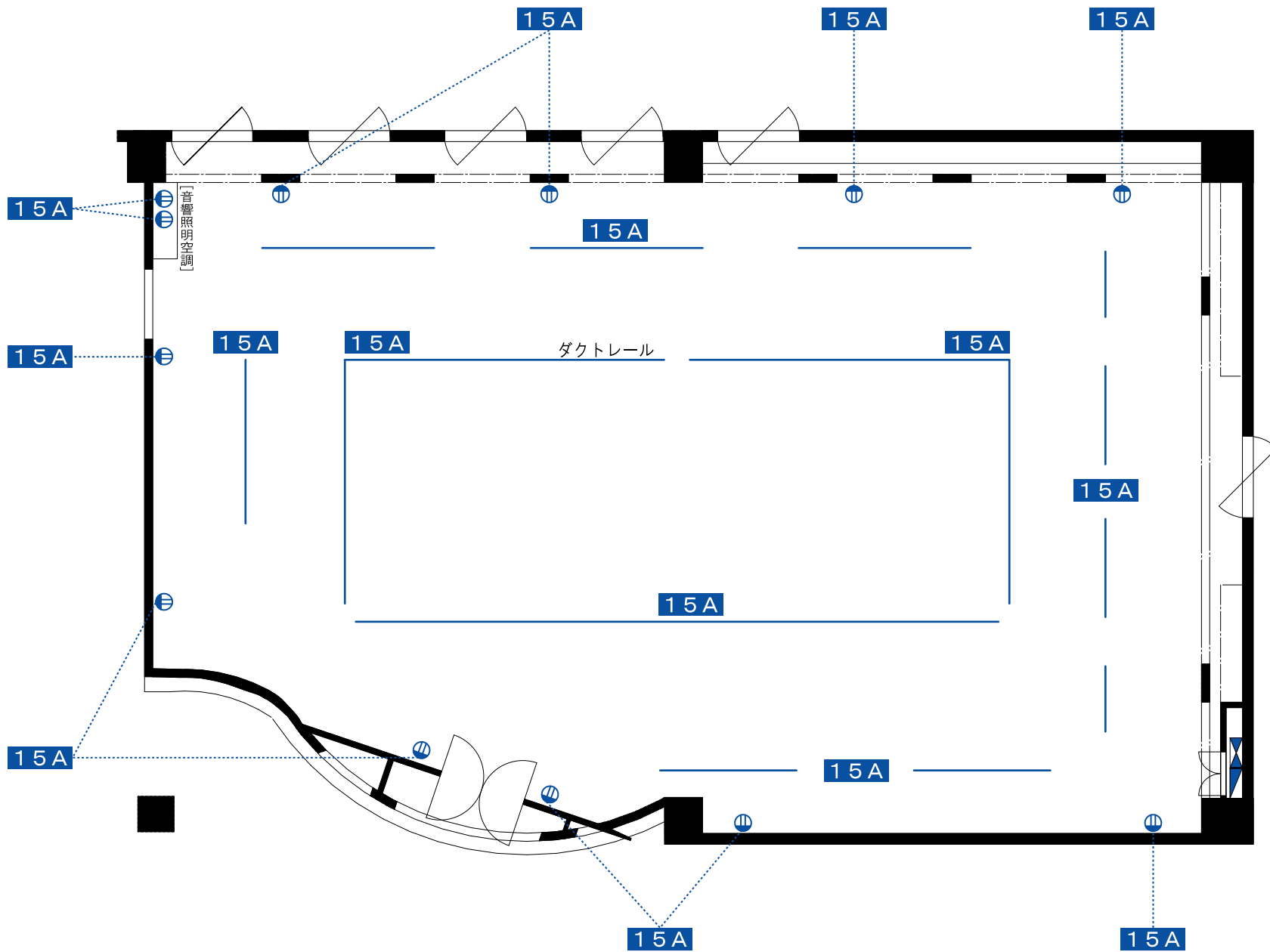
■ Bホール 〈電気回路図〉
